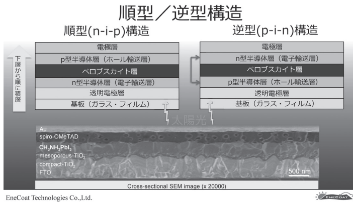
図1 ペロブスカイト積層断面図
